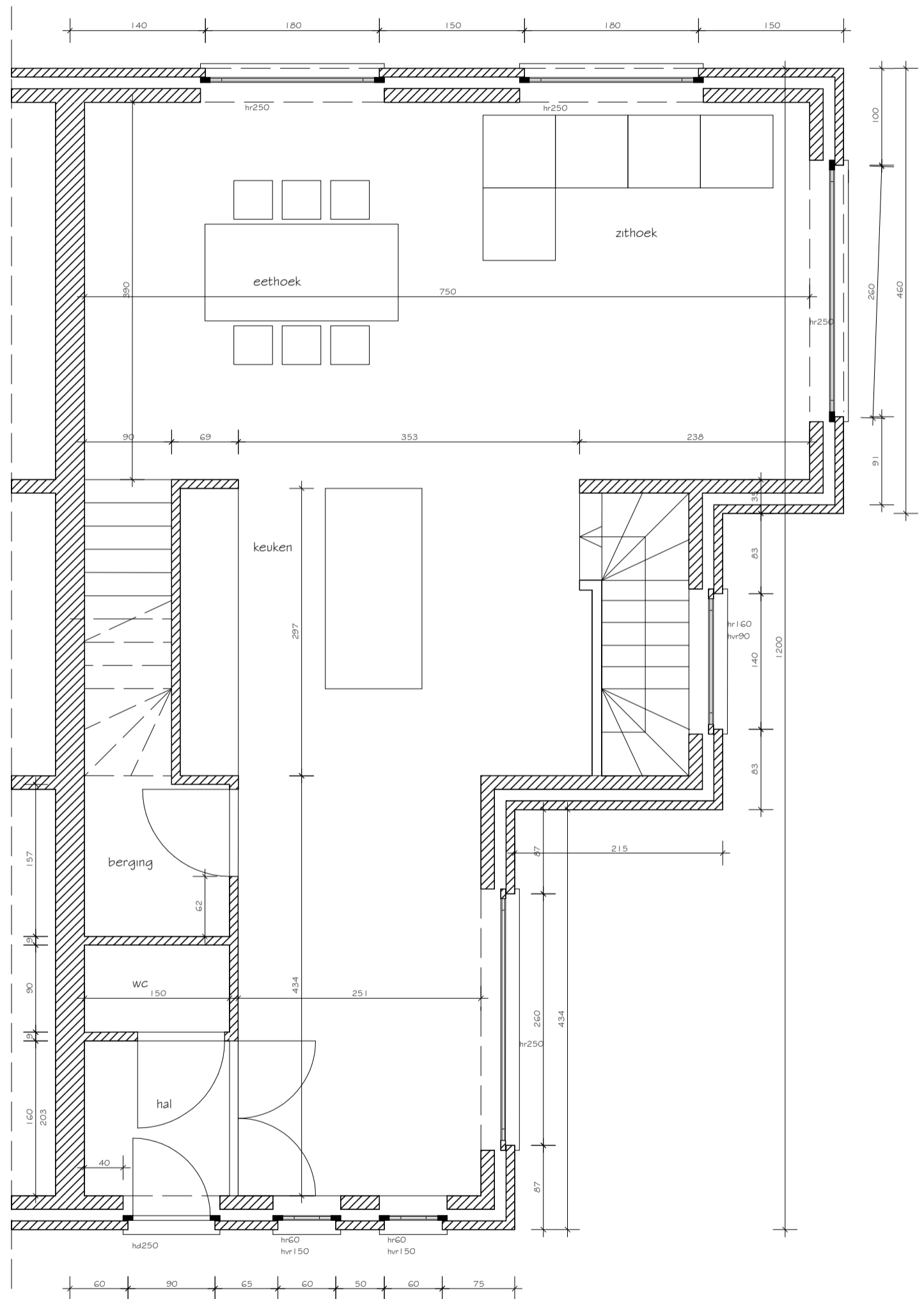
WONING 9 gelijkvloers
